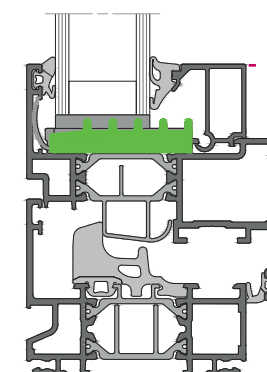
Fenêtre OV HI+
